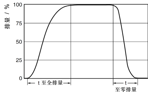
流量控制的动态特性*
