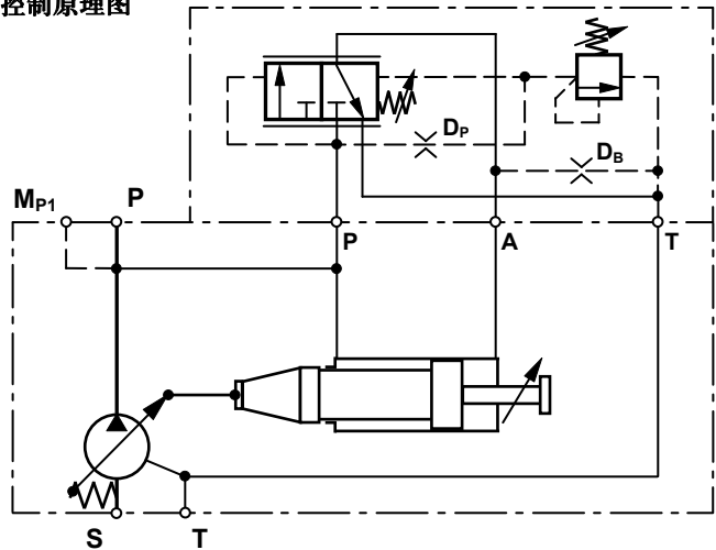
控制原理图
