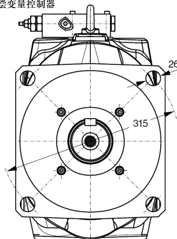
X向视图
