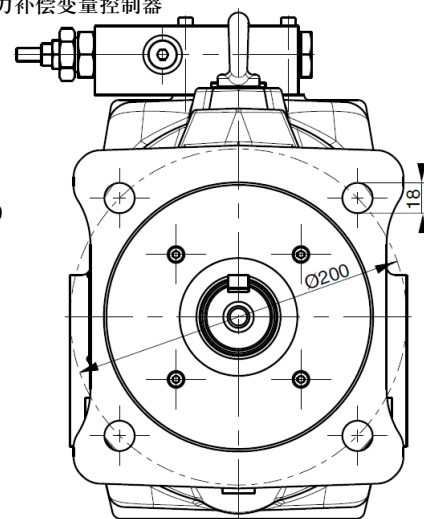
X向视图
