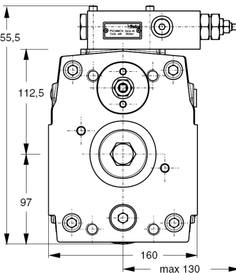
X向视图
