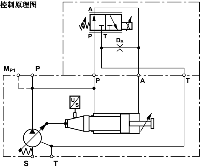
控制原理图
