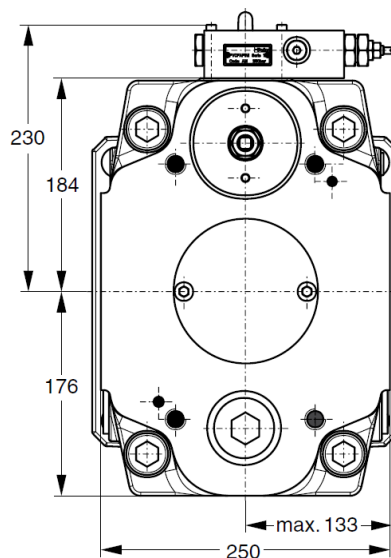
X向视图
